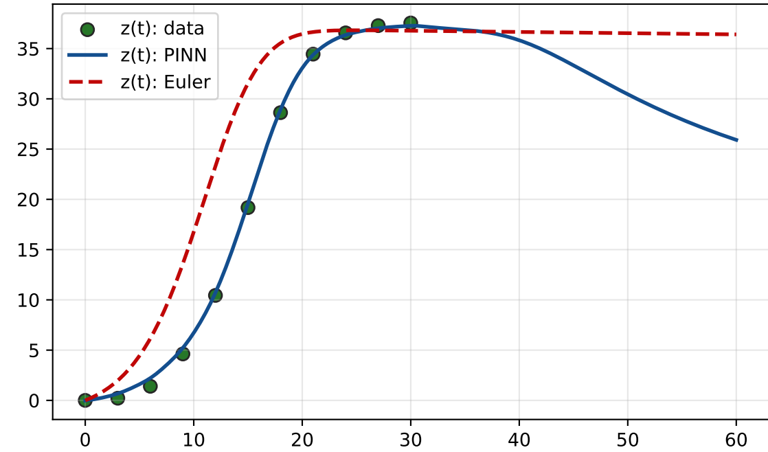
z(t): Ethanol
